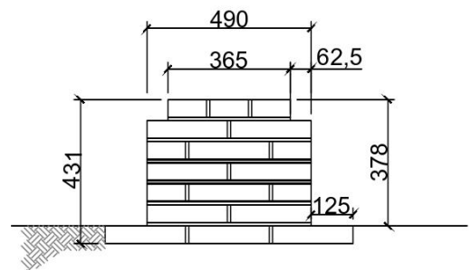
景墙立面图
